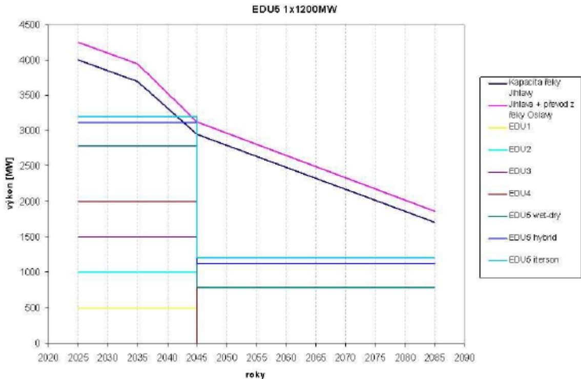
Graf č. 21 Kapacita řeky Jihlava potřebná k provozu jednotlivých bloků EDU (podle výkonu)
