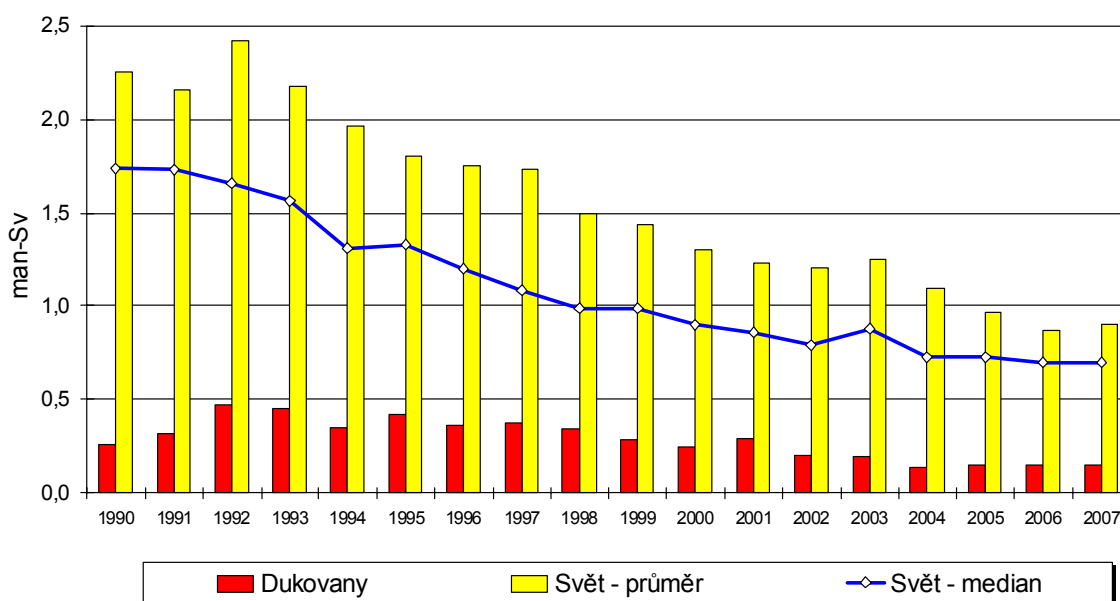
Obr. č. 3.4. Kolektivní efektivní dávka (ozáření pracovníků v kontrolovaném pásmu)
