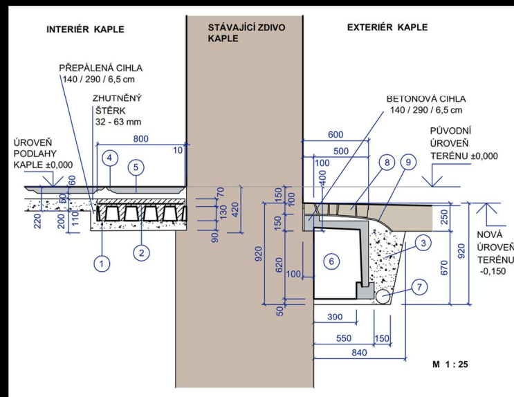
Spodní stavba kaple
