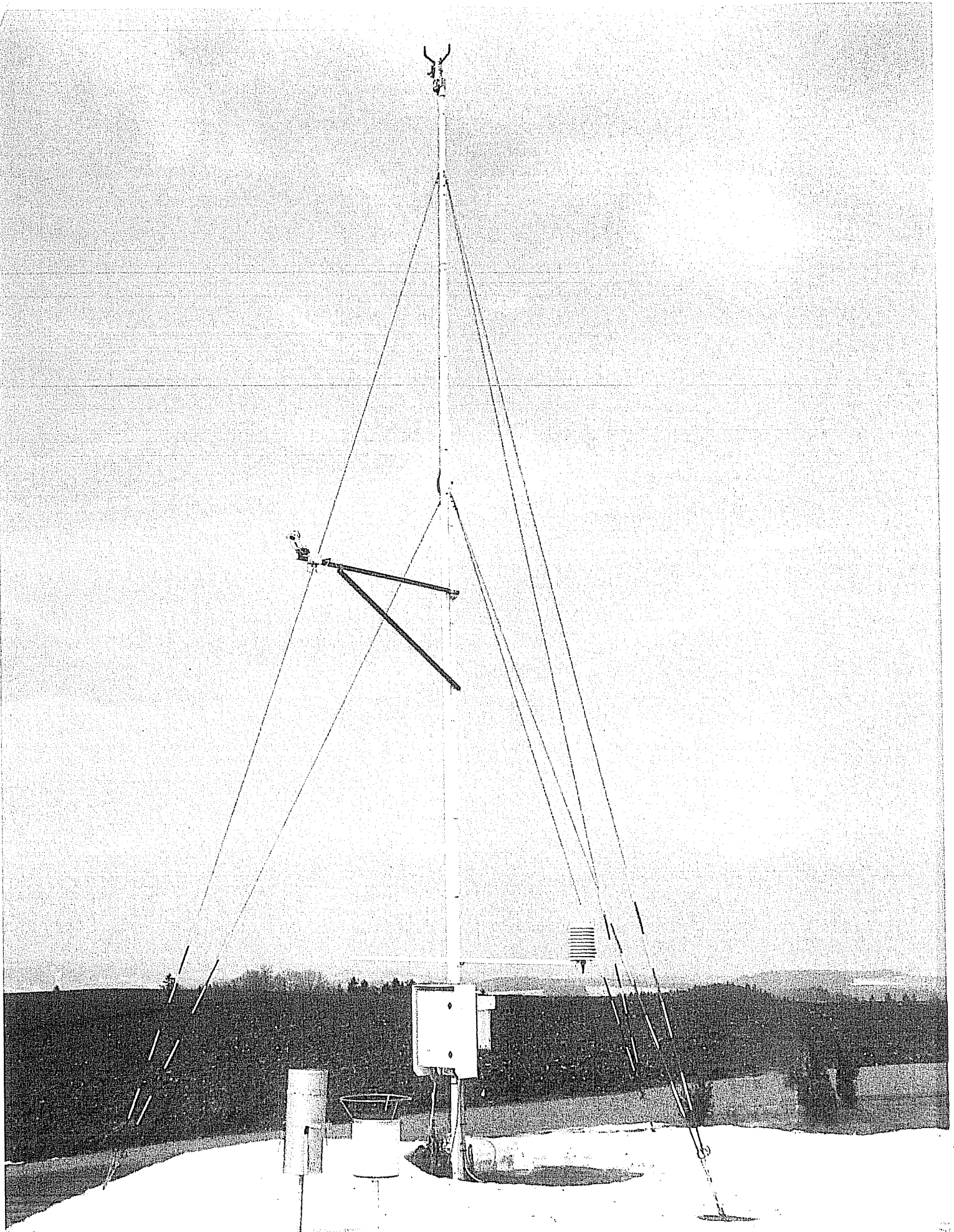
Obr. Vzor automatizované meteorologické stanice v terénu.
