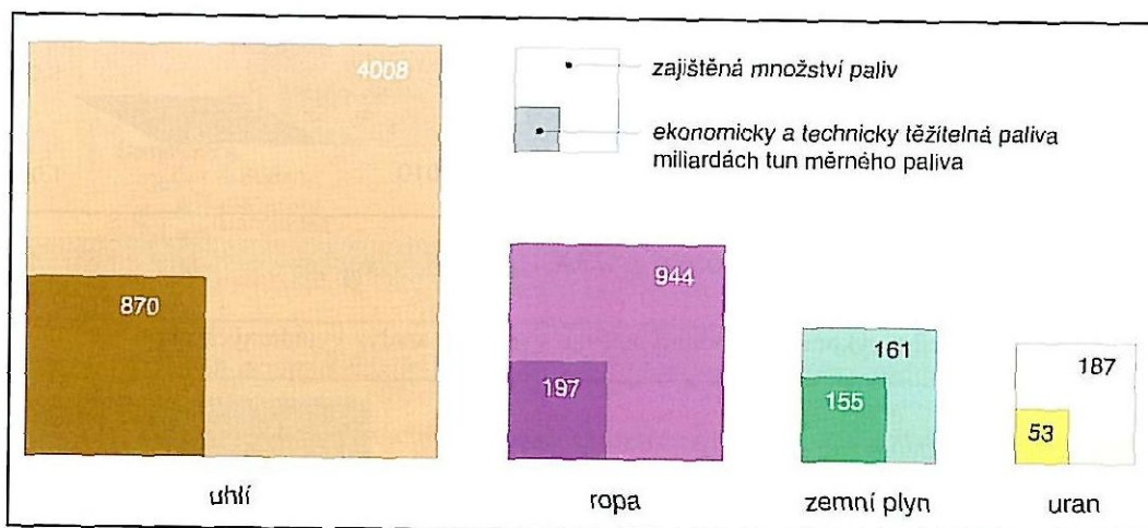
Obr. 7. Světové zásoby a rezervy paliv.
