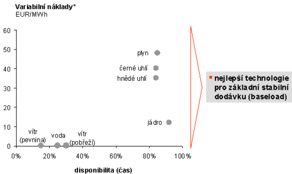
Obr. č. 1.4. Porovnání efektivity zdrojů
