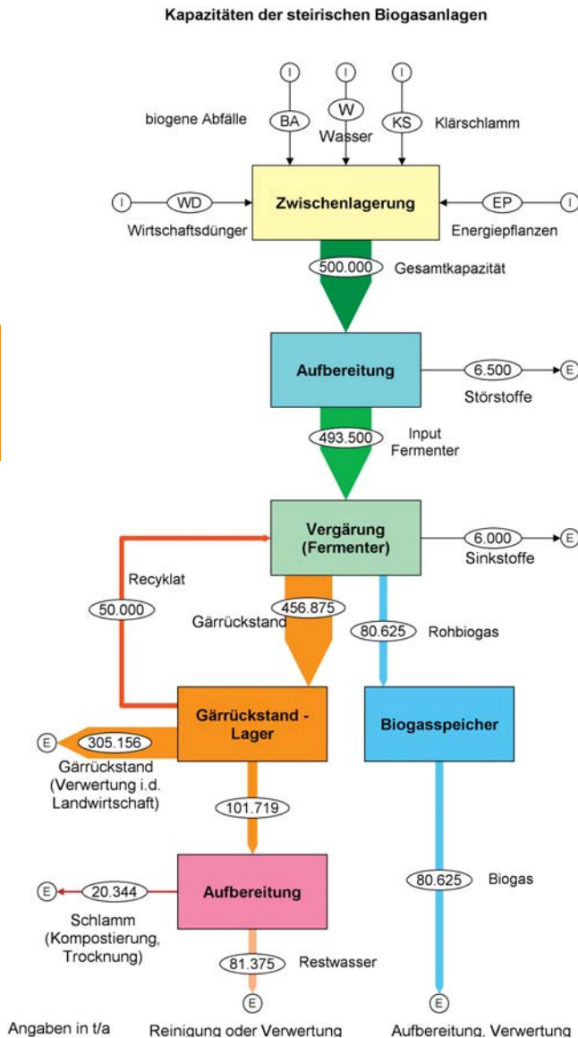
Abbildung 47: Kapazitäten der steirischen Biogasanlagen und Stoffflussdarstellung
