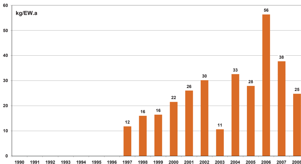
Abbildung 73: Kommunal gesammelten Mengen an Baurestmassen in der Steiermark 1999-2008
