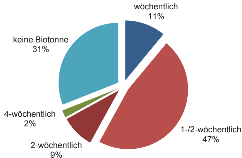
Abbildung 41: Abfuhrintervalle im Bereich Bioabfallsammlung in der Steiermark (Erhebung bei 117 Gemeinden)
