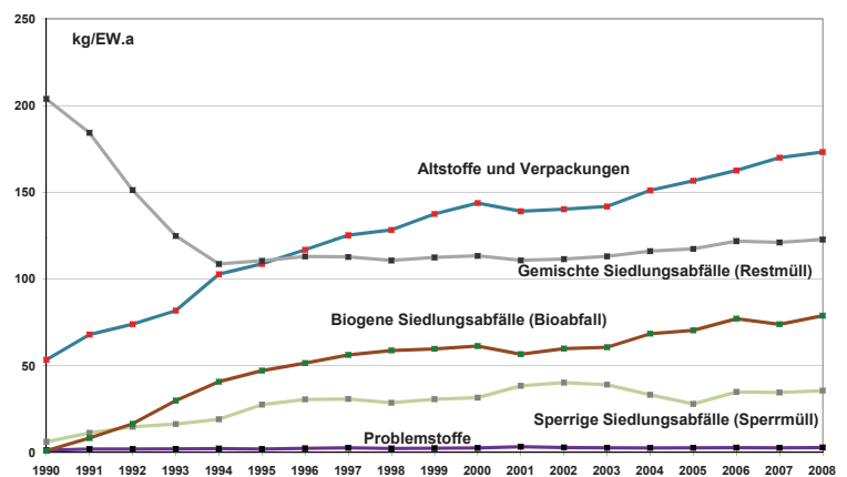
Entwicklung des kommunalen Abfallaufkommens in der Steiermark (ohne Elektro- und Elektronikaltgeräte und Straßenkehricht)
