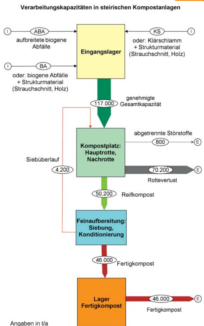
Abbildung 44: Kapazitäten der steirischen Kompostieranlagen und Stoffflussdarstellung
