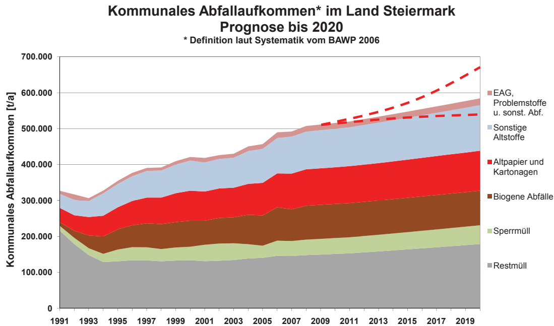
Abbildung 78: Abfallmengenprognose für das Land Steiermark (Szenario „Trend mit 1% realem Wirtschaftswachstum“) Quelle: Beigl & Lebersorger, 2010
