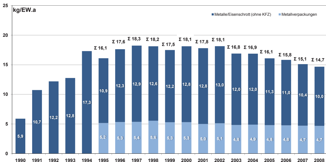
Abbildung 55: Kommunale Sammelmengen von Metallverpackungen und Altmetallen/Eisenschrott (Altstoffe) in der Steiermark 1990 bis 2008
