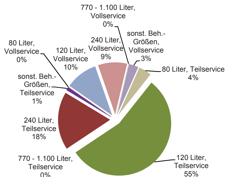
Abbildung 40: Behälterverteilung im Bereich Bioabfallsammlung in der Steiermark (Erhebung bei 117 Gemeinden)
