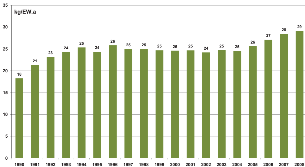
Abbildung 51: Kommunale Sammelmengen von Altglas (Verpackungen) in der Steiermark 1990 bis 2008
