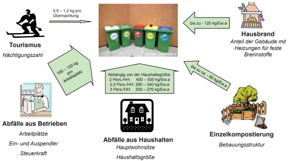
Abbildung 14: Einflussfaktoren auf die kommunalen Abfallsammelmengen (Quelle: Beigl & Lebersorger, 2010)
