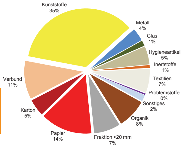
Abbildung 19: Zusammensetzung des Restmülls (Volumen-%) im Jahr 2008 129
