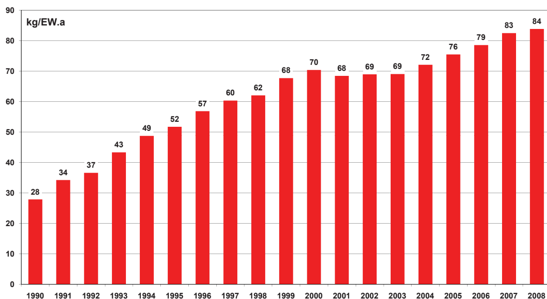
Abbildung 48: Kommunale Sammelmengen von Altpapier in der Steiermark 1990 – 2008.
