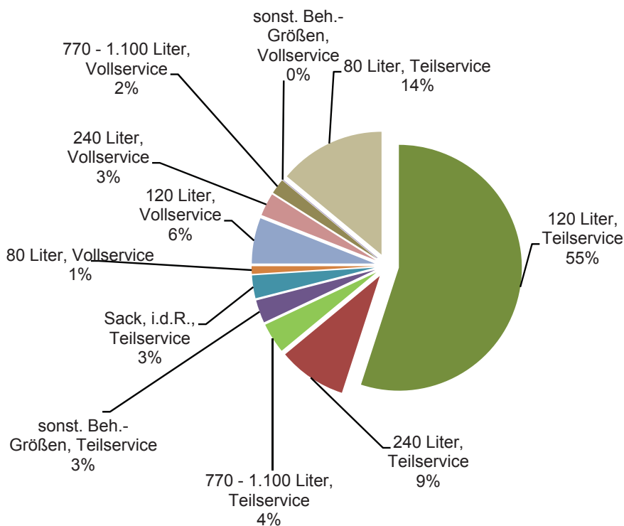
Abbildung 17: Behälterverteilung bei der Restmüllsammlung in steirischen Gemeinden (Erhebung bei 117 Gemeinden)
