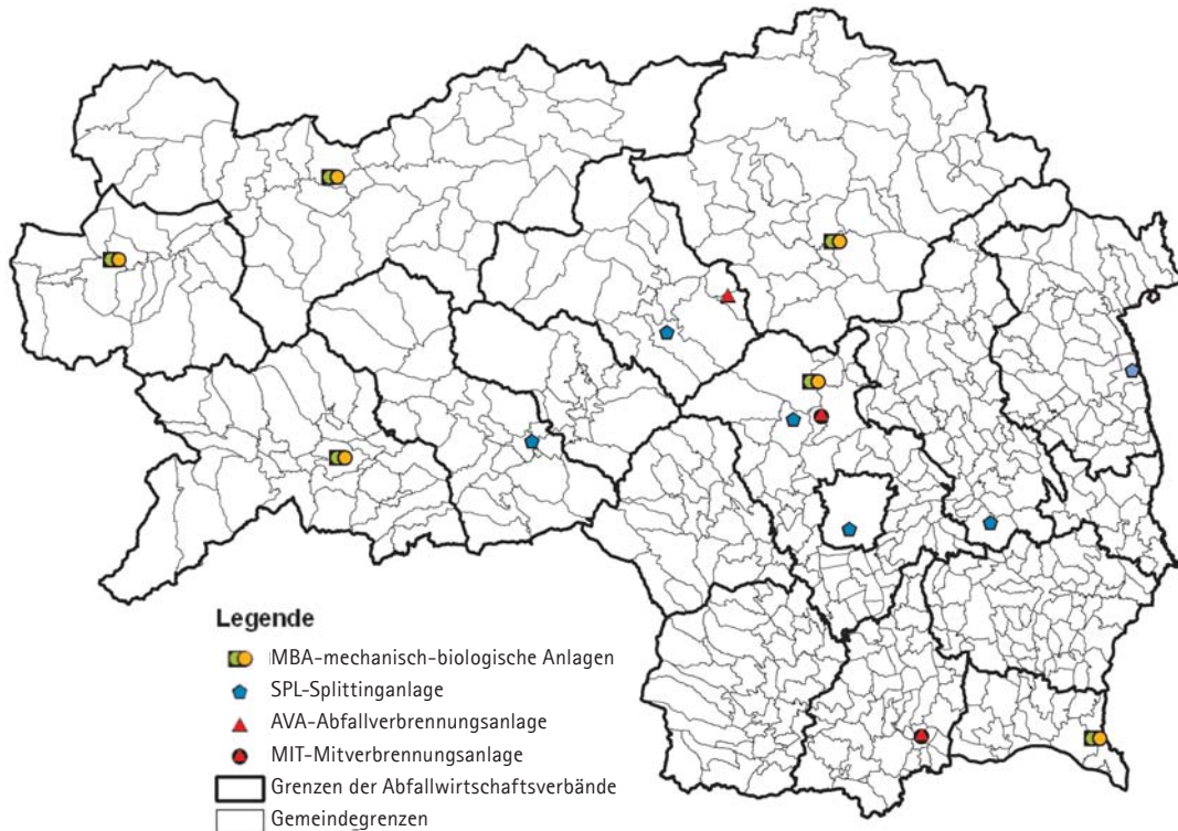
Abbildung 24: Standorte zur Behandlung von u.a. gemischten Siedlungsabfällen (Restmüll) in der Steiermark: mechanisch-biologische Abfallbehandlungsanlagen (MBA), Restmüllsplittingsanlagen, Verbrennungs- und Mitverbrennungsanlagen, Stand 1.1.2009.
