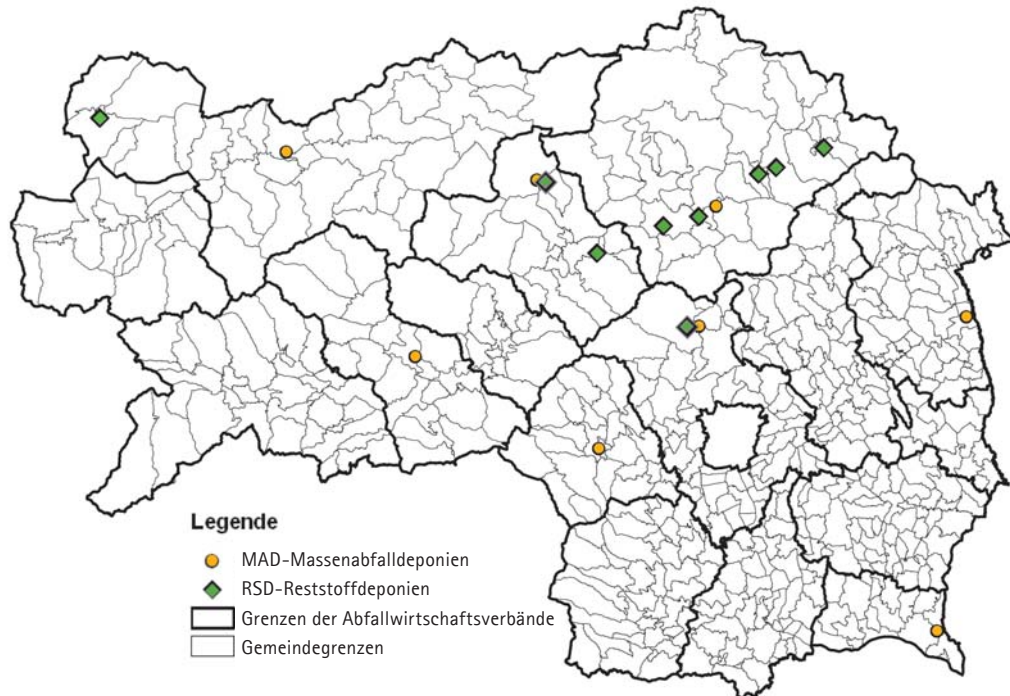
Abbildung 27: Standorte der Massenabfall- und Reststoffdeponien in der Steiermark, Stand 1.1.2009
