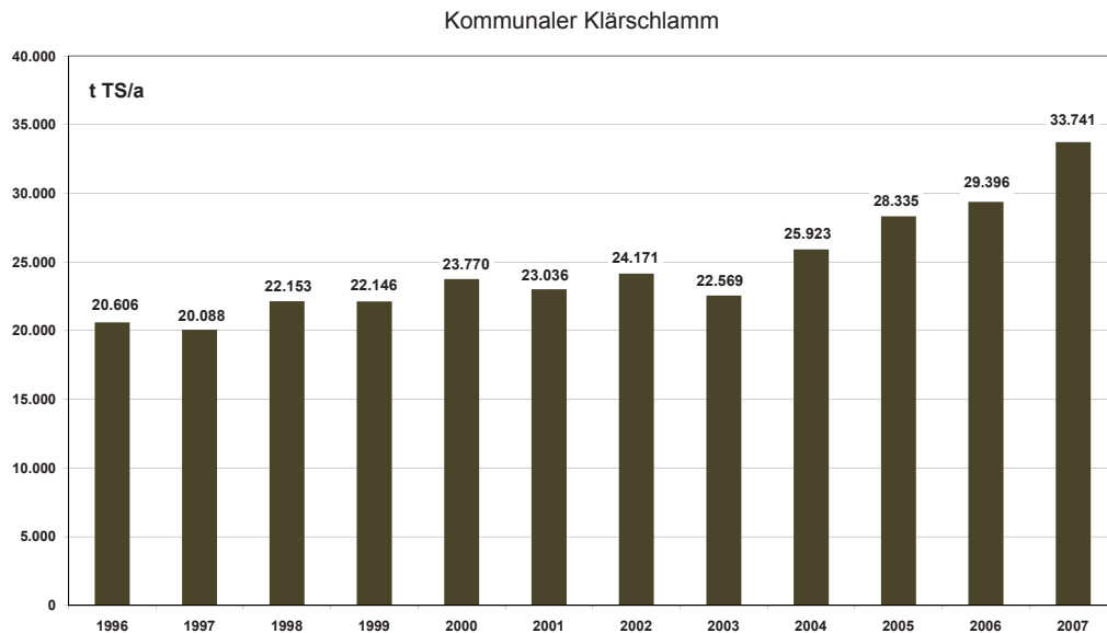
Abbildung 70: Kommunales Klärschlamm aufkommen in der Steiermark 1996 – 2007
