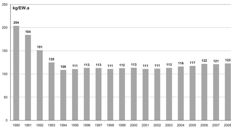
Abbildung 15: Entwicklung der kommunalen Sammelmenge pro EinwohnerIn in der Steiermark im Zeitraum 1990 – 2008 für gemischte Siedlungsabfälle. Der starke Rückgang der Sammelmengen im Zeitraum 1990 – 1994 ist auf die flächendeckende Etablierung der getrennten Sammlung von Biomüll, Altstoffen und Verpackungen zurückzuführen.
