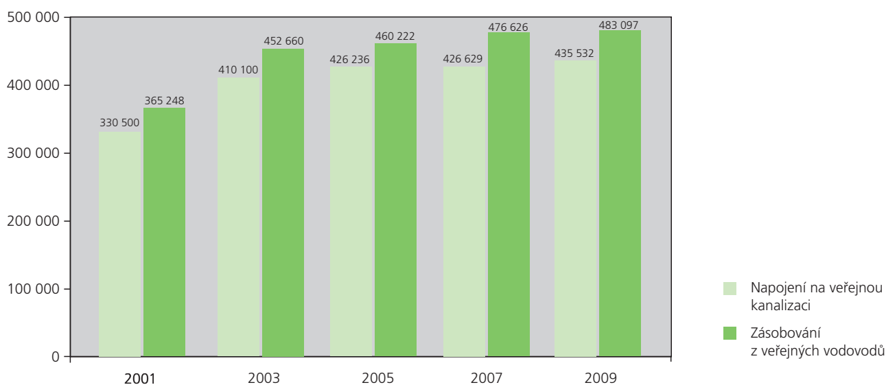
Vývoj počtu obyvatel kraje Vysočina zásobovaných z veřejných vodovodů a napojených na veřejnou kanalizaci od roku 2001 do roku 2009
