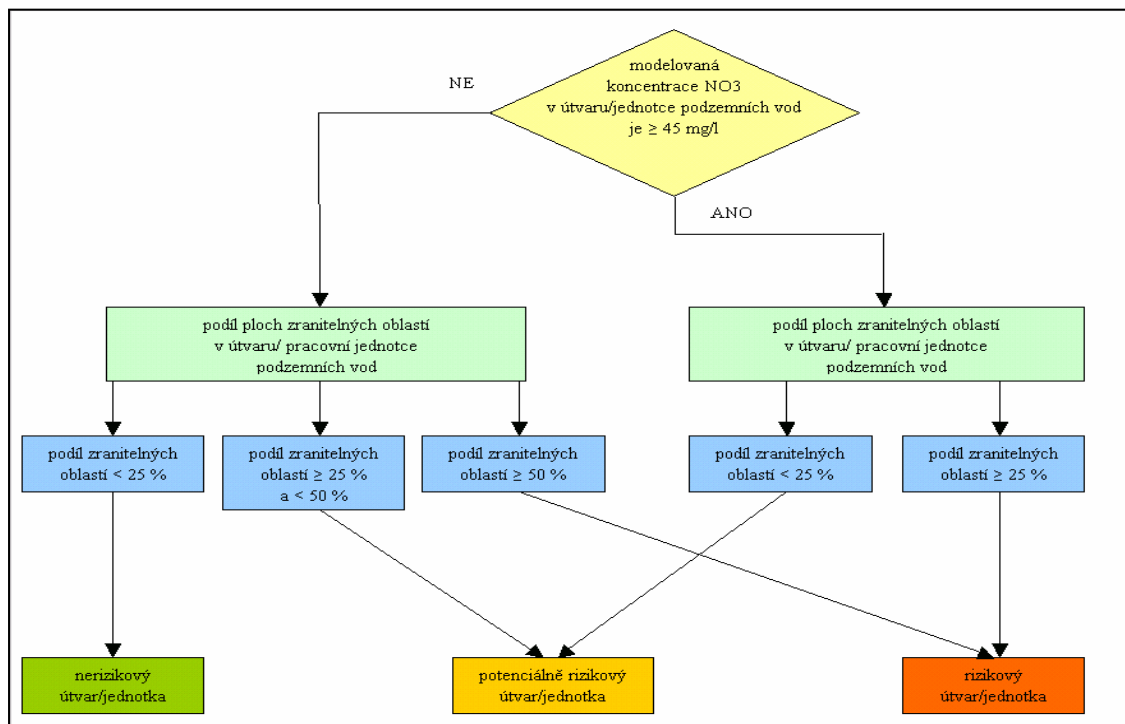
Obr. B.7 – Schéma hodnocení rizikosti útvarů podzemních vod nebo pracovních jednotek z pohledu plošného znečištění vod dusíkem
