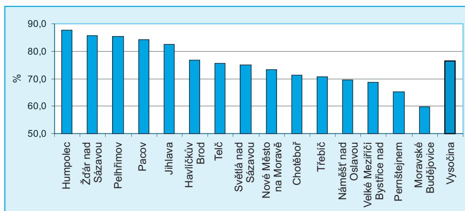
Obr. 2: Sídla kraje Vysočina, která jsou napojena na čistírnu odpadních vod nebo jsou navržena na napojení na čistírnu odpadních vod
