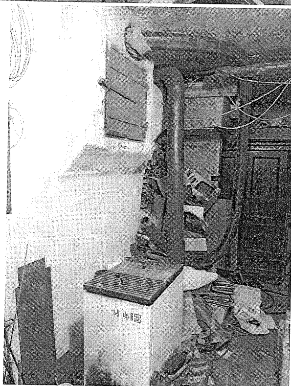
fotodokumentace stávajícího kotle s napojením na otopnou soustavu a odkouření
