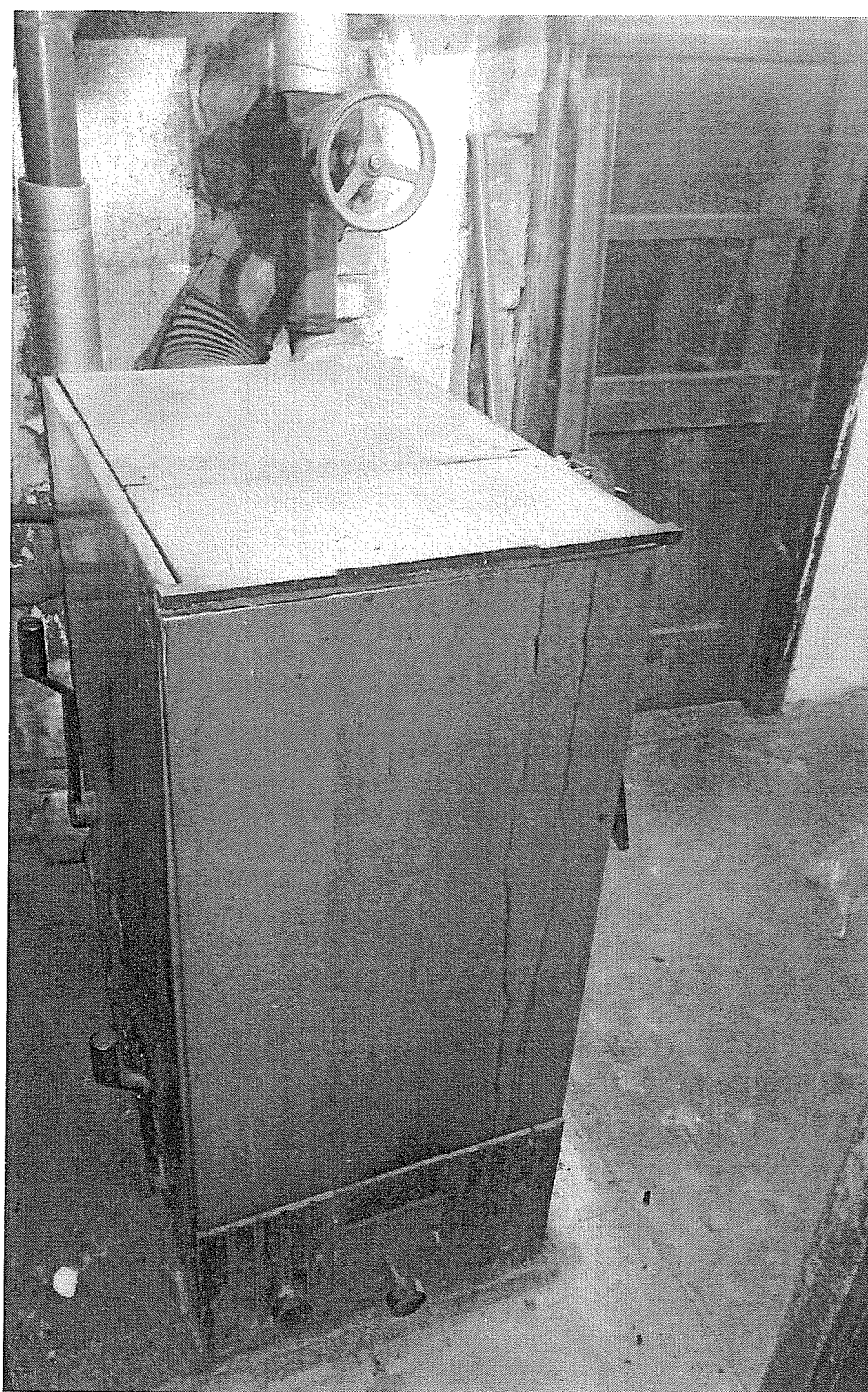
Teplovodní kotel DS - 25
