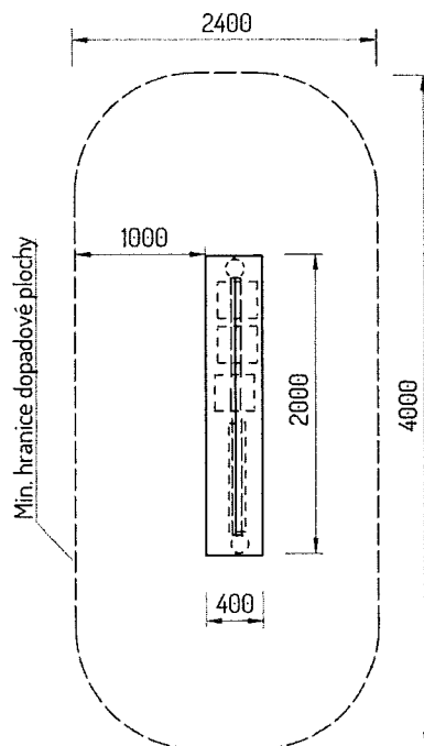
Půdorys tabule s vyměnitelnými panely
