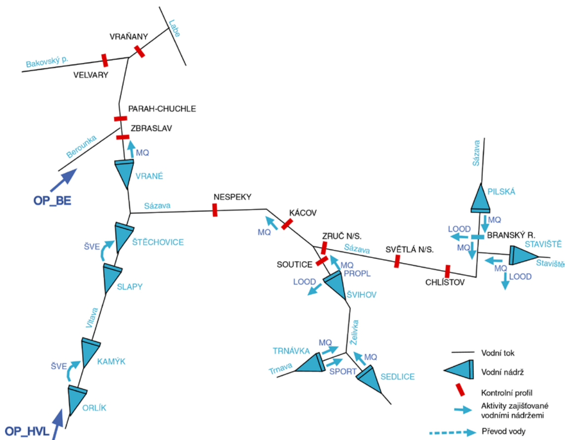
Obr. č.5 - Výpočtové schéma vodohospodářské soustavy
